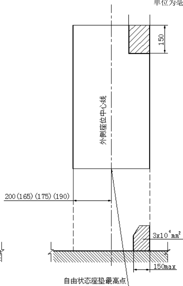
图10 外侧座椅空间的允许侵入
