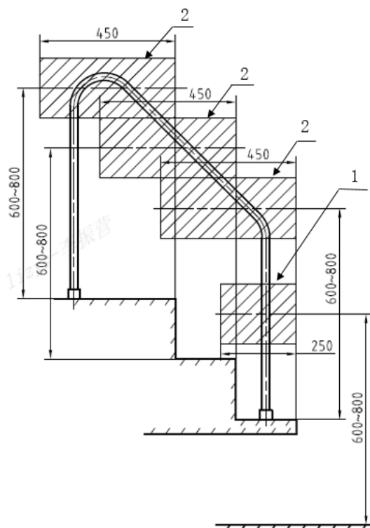
图 11 低扶手位置示意图
