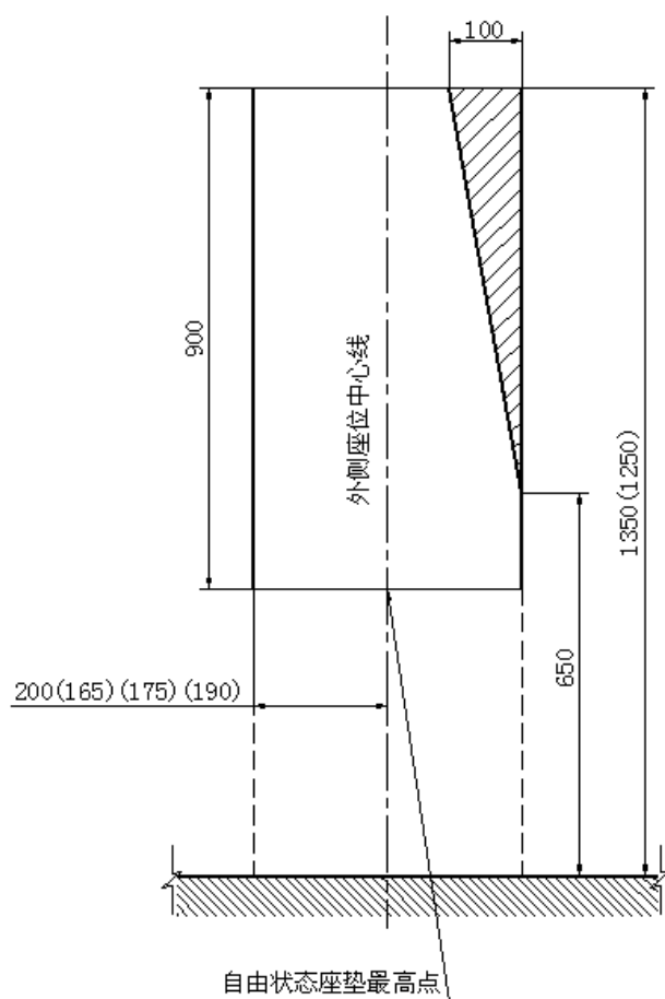
图9 座椅上方的自由空间
