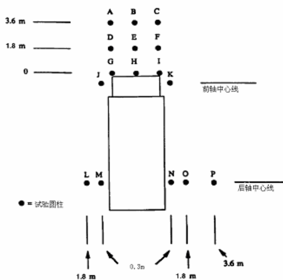
图C.1 视野检验中检验圆柱体的位置
