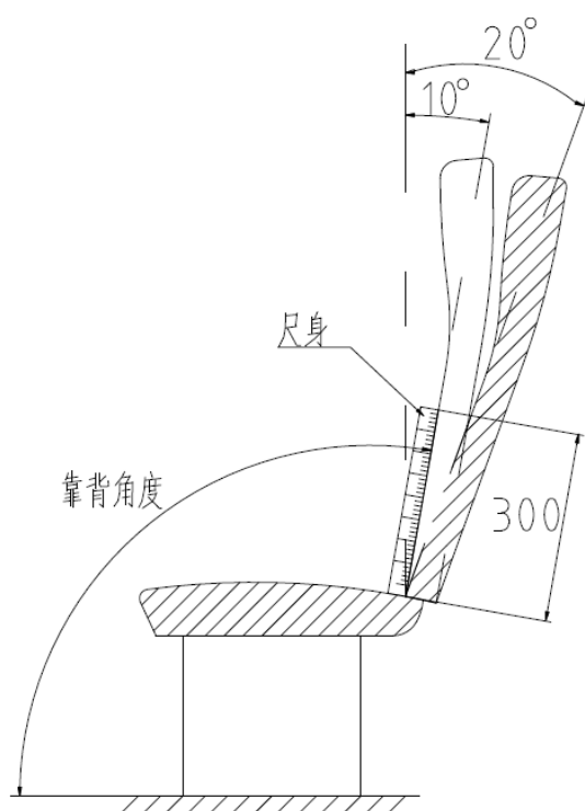
图6 座椅靠背角度测量方法示意图
