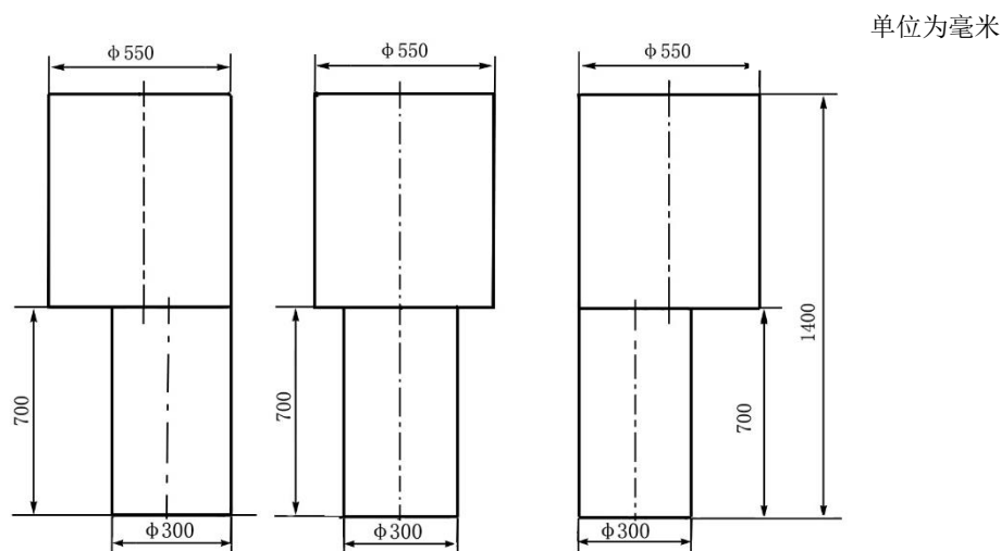
图4 应急门引道测量装置
